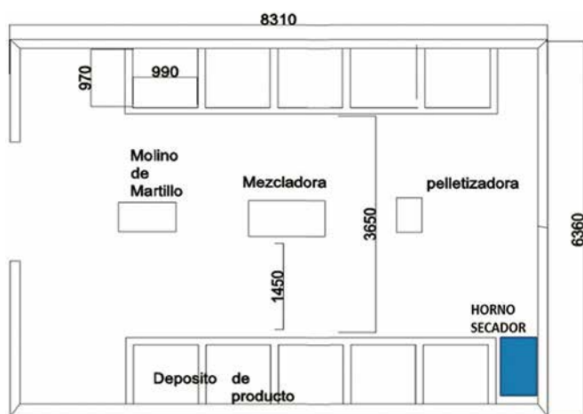
Figura 1. Distribución espacial de equipos y área requerida para la unidad modelo artesanal de elaboración de alimento para uso animal.
